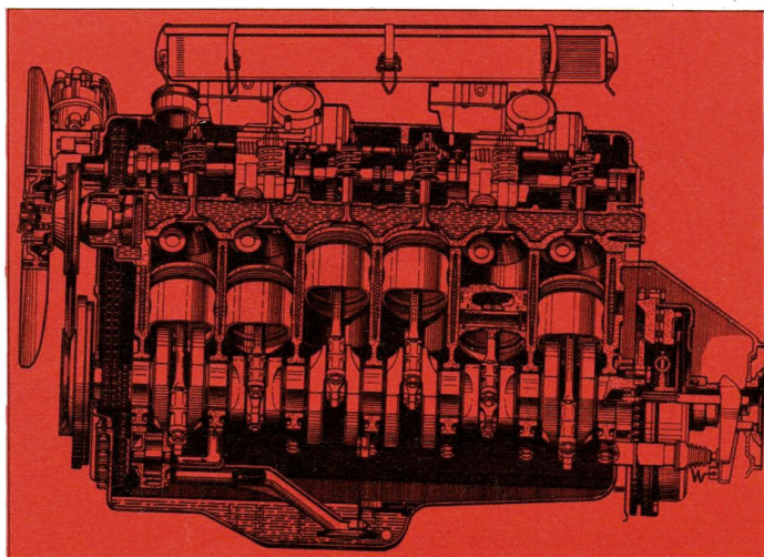
Der Motorquerschnitt
