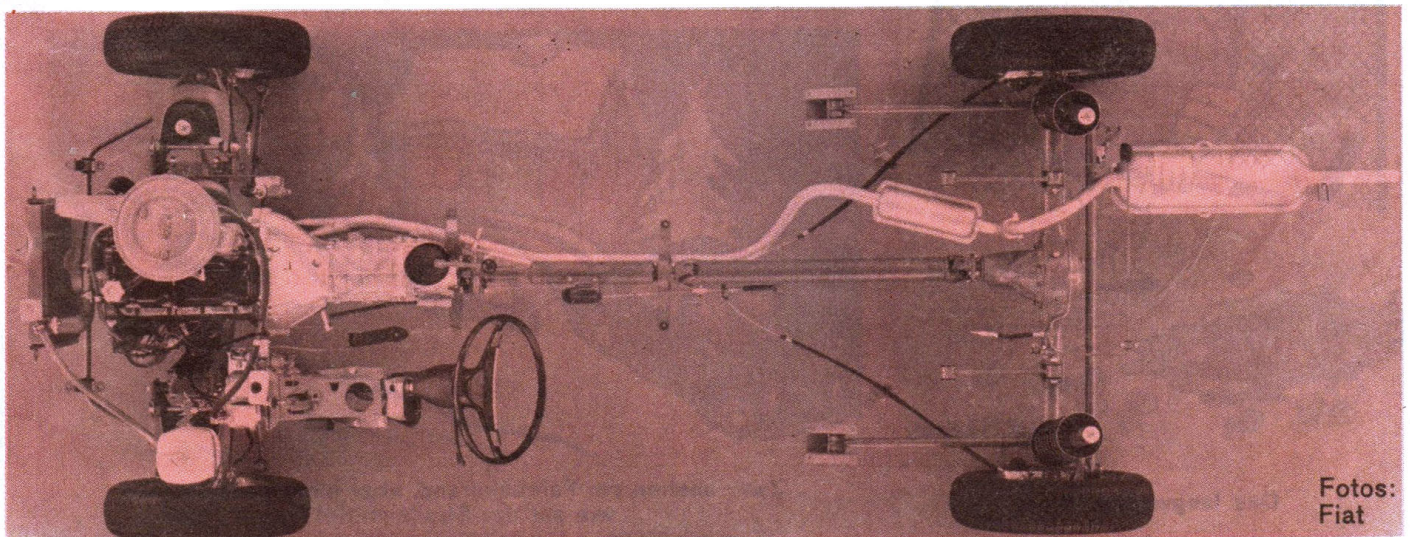
Die mechanischen Organe des 124 Special
